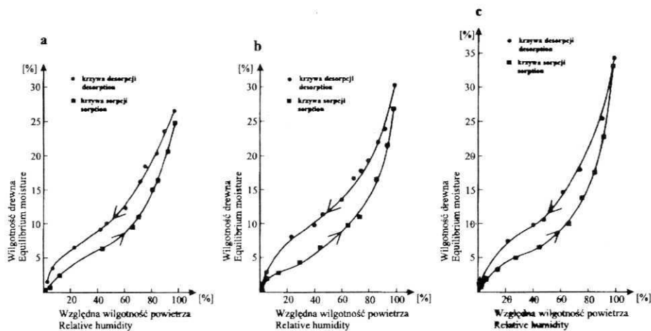
Rys. 1. Krzywe sorpcji i desorpcji drewna bielu sosny:
