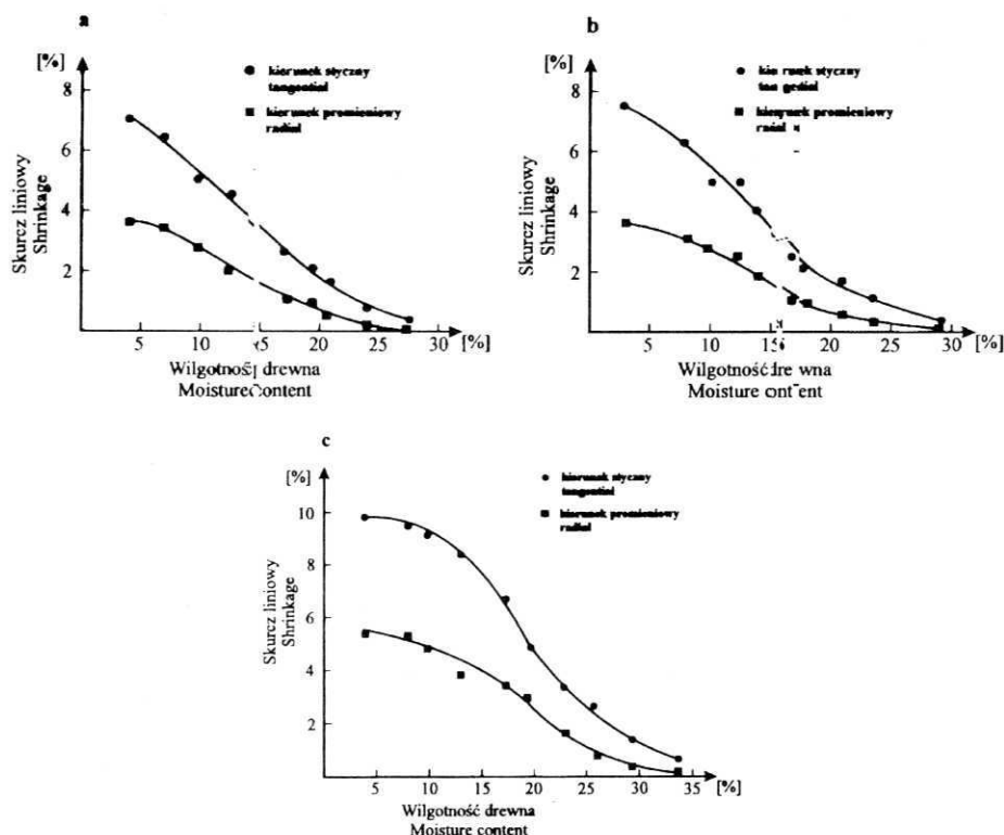
Rys. 3. Krzywe skurczu drewna biału sosny: a - nie ekstrahowanego, b - po wyodrębnieniu substancji ekstrakcyjnych, c - po wyodrębnieniu hemiceluloz
